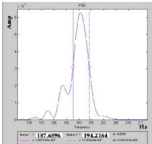
图 8: 低频半峰宽
