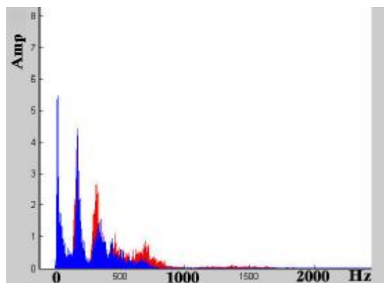
图 5：发声频谱
