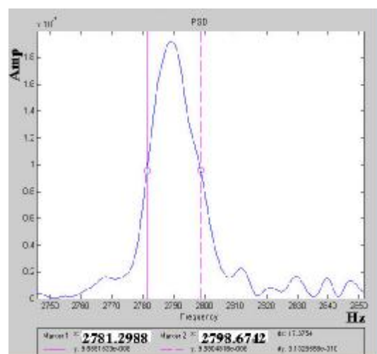
图 9: 高频半峰宽
