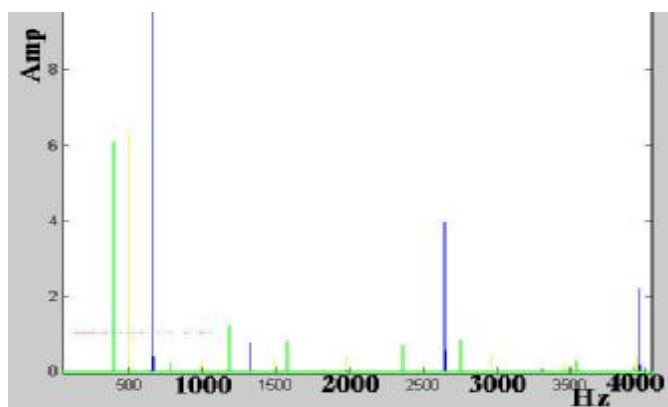
图 11: 定音器频谱
