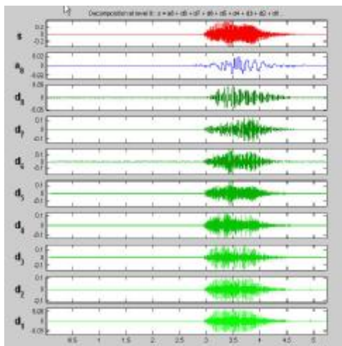
图 13 小波分解系数图
