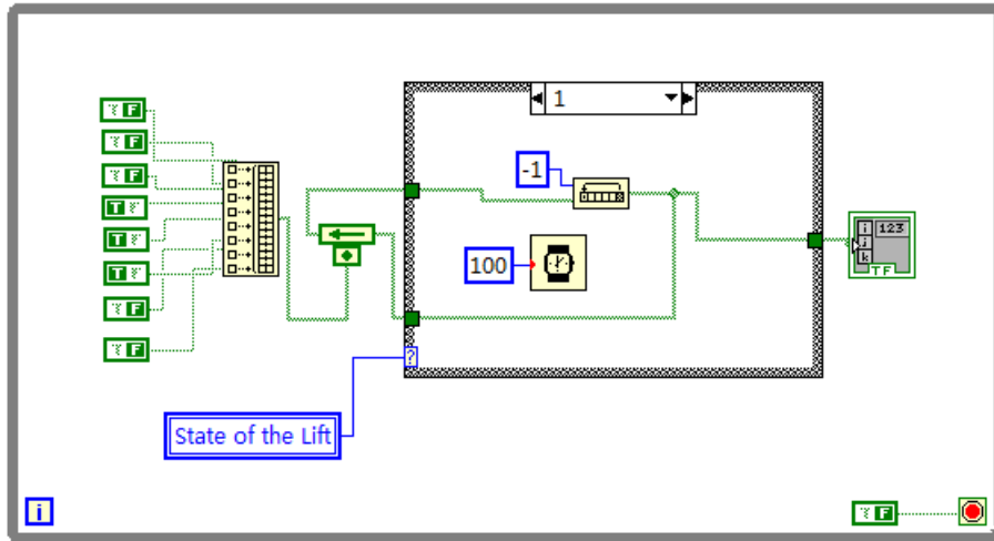
图 (5): 电梯操控系统的后台程序 4
