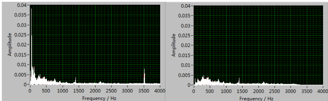
图 2.6 滤波前后声音信号频谱图
