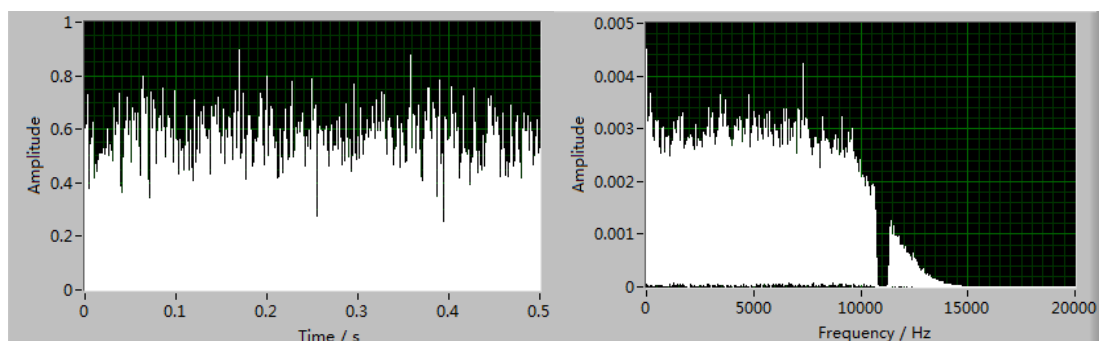
图 2.3 白噪音信号的声音强度和频率分布
