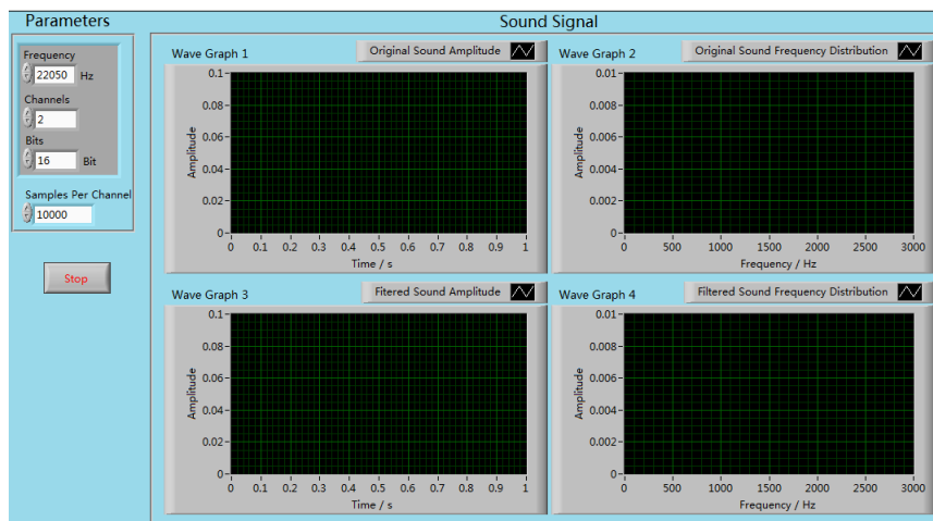
图 2.1 程序前面板
