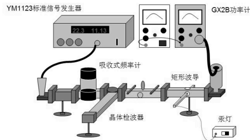
图3.实验装置简图
