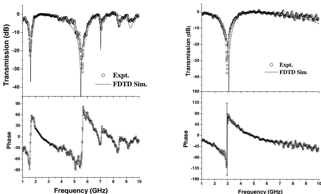
图 2（左）16mm 第一级长度四级分形板，电场 x 方向偏振时透射与相位谱线。 （右）电场 y 方向偏振时透射与相位谱线。圆点为实验点，实线为模拟数据。
