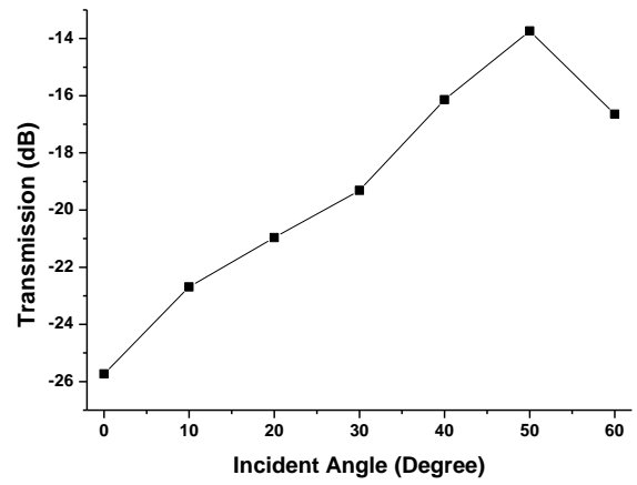
图7 (左)16mm 四级分形板不同入射角入射时的透射谱线, (右) 在 1.56GHz 处透射率与入射角的关系
