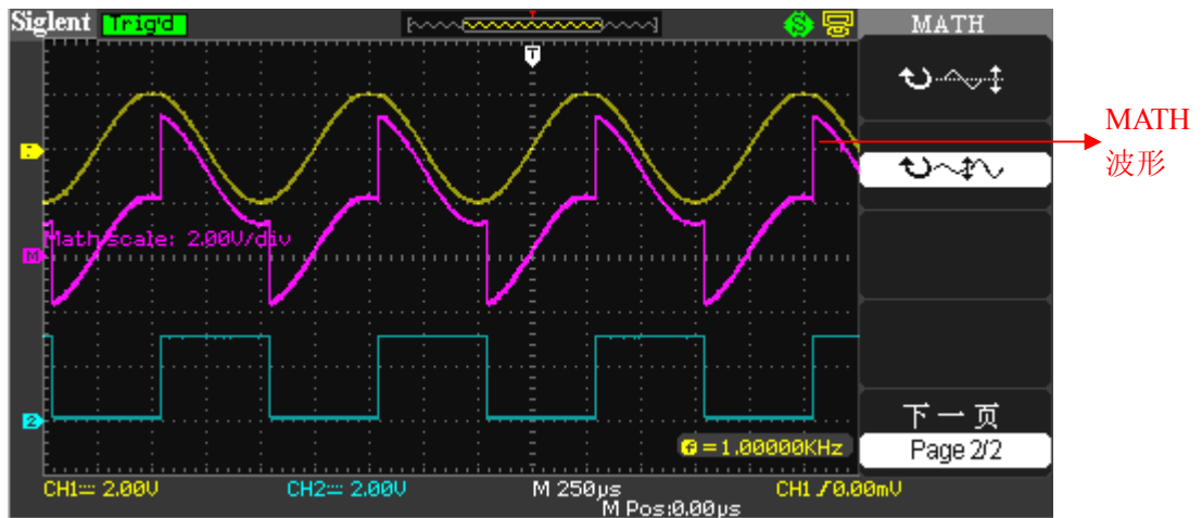
图 2-12 CH1 与 CH2 的波形相加
