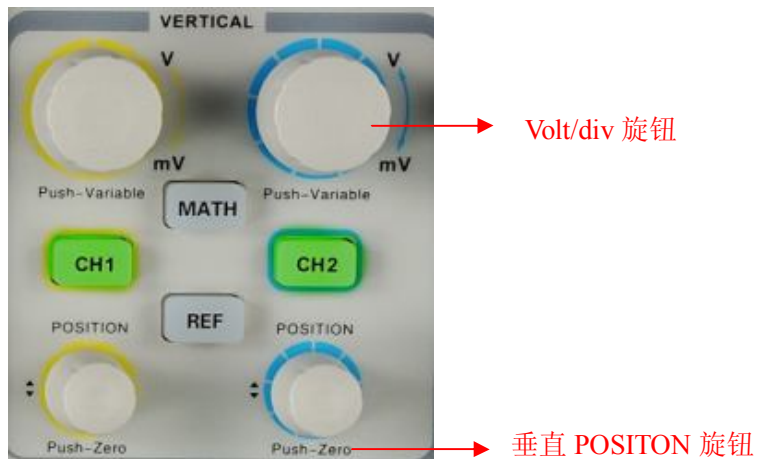
图 2-5 垂直系统
