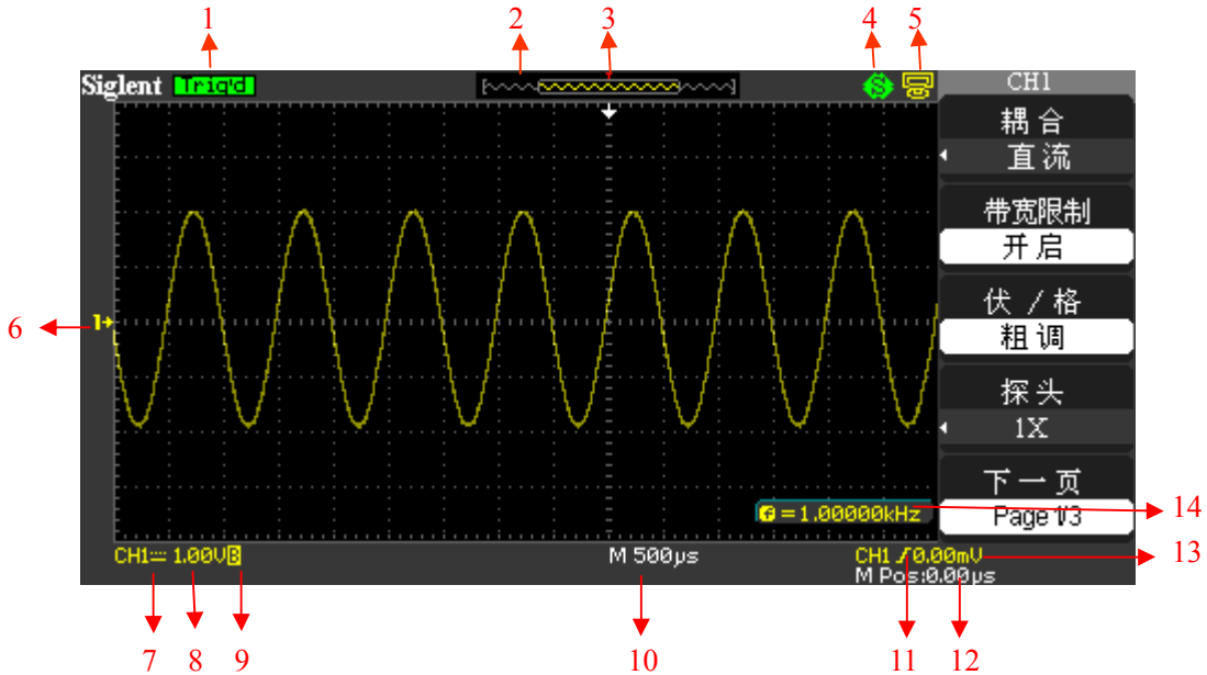
图 1-2 SDS1000CML 界面显示区
