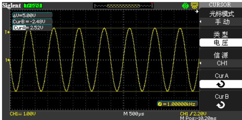
图 2-44 手动测量
