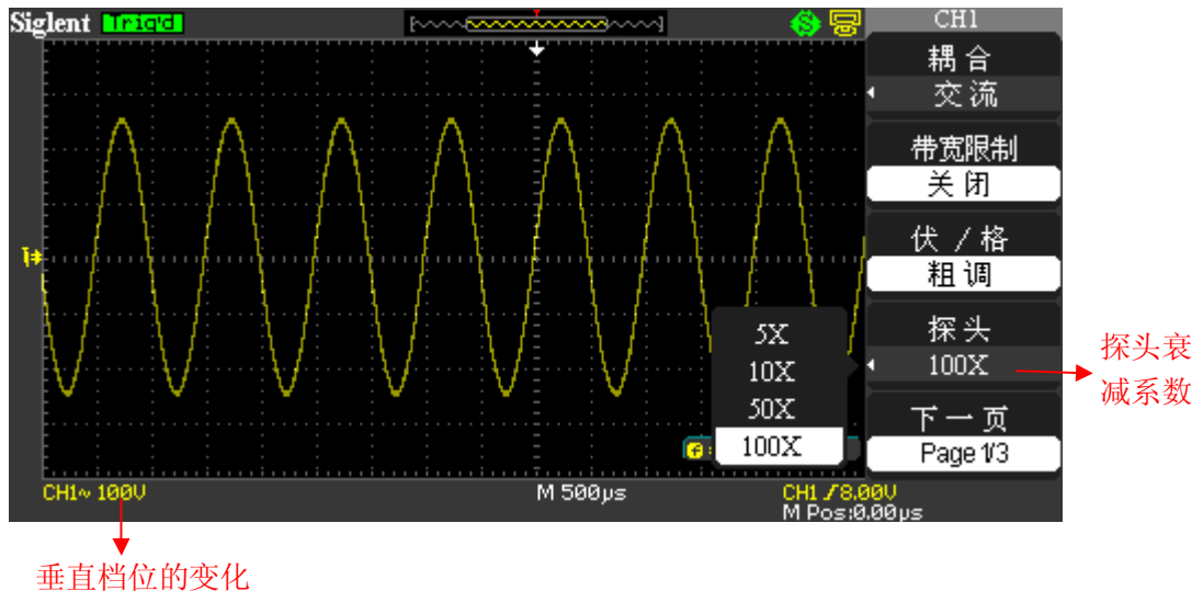
图 2-9 探头比例设置
