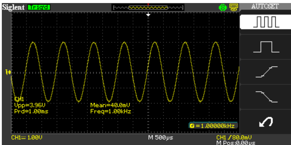
图 2-3 自动设置
