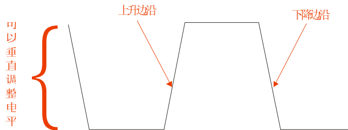
图 2-29 斜率和电平
