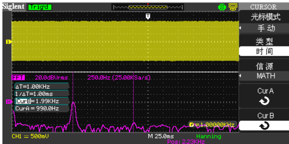
图 2-15 测定 FFT 频谱
