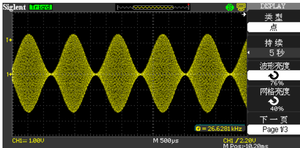
图 2-42 利用持续选项观察调幅波
