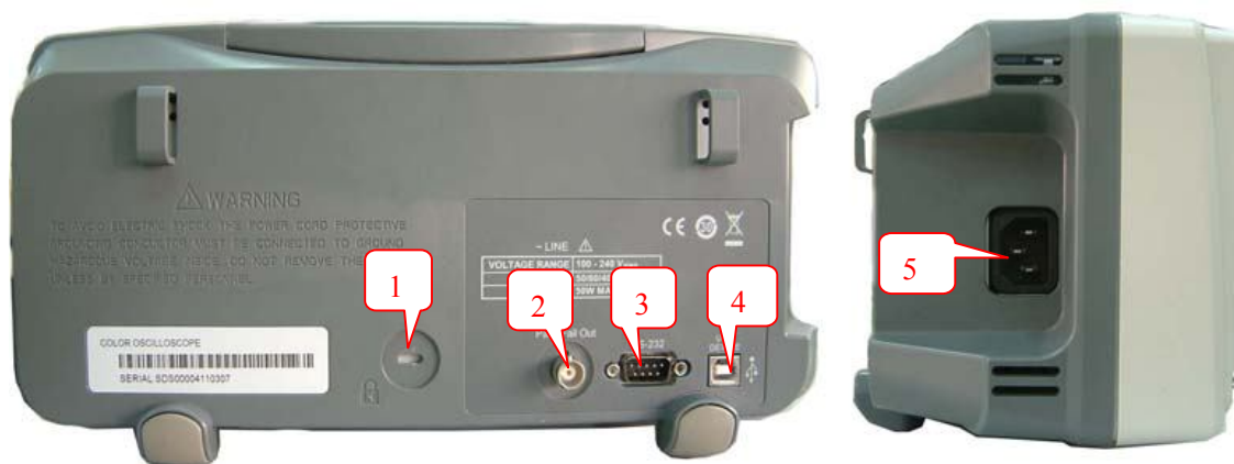
图 1-3 SDS1000CML 背部接口
