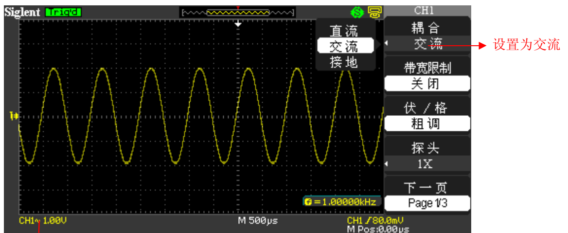
图 2-6 通道耦合设置
