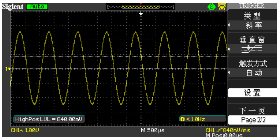
图 2-27 斜率触发功能菜单 2
