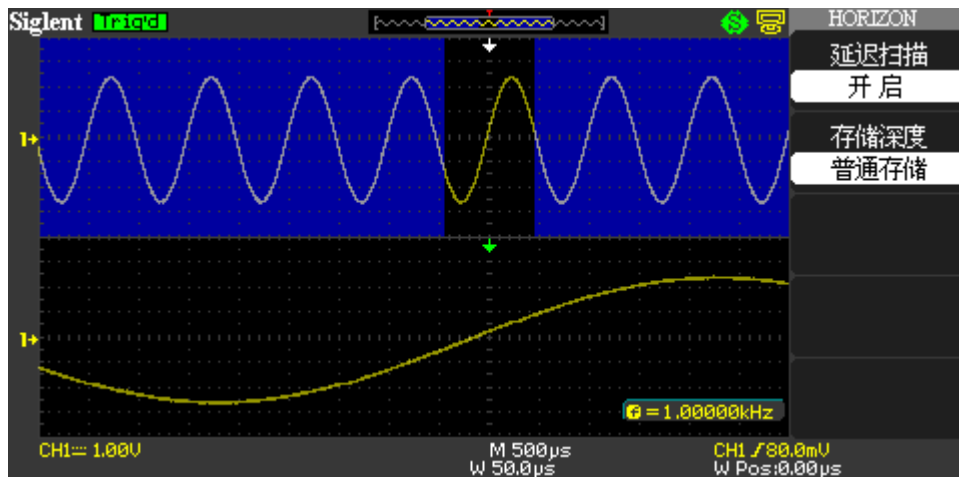
图 2-19 HORI MENU 菜单
