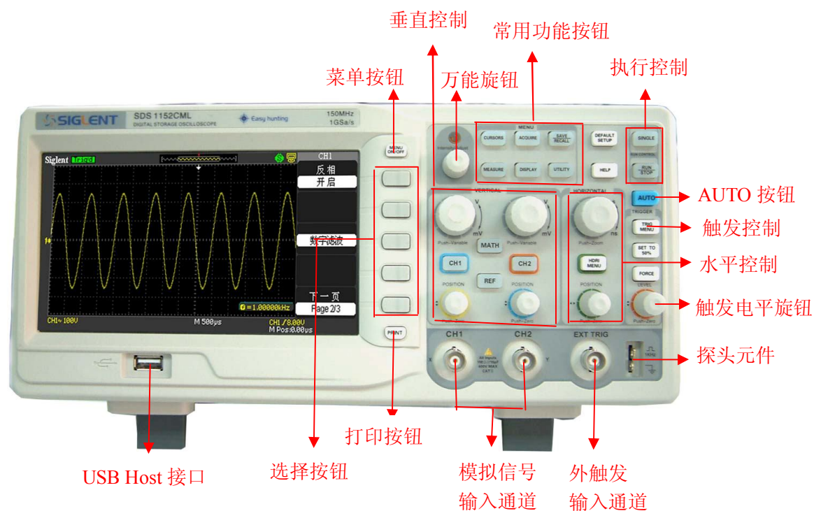
图 1-1 SDS1000CML 前面板
