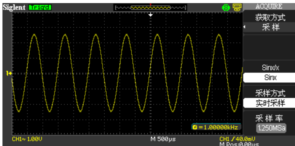
图 2-32 采样模式
