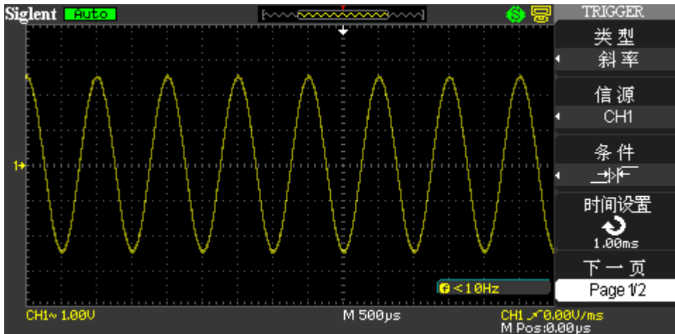
图 2-26 斜率触发功能菜单 1
