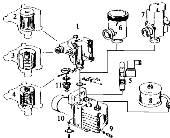
图 2 改造部件安装位置图
