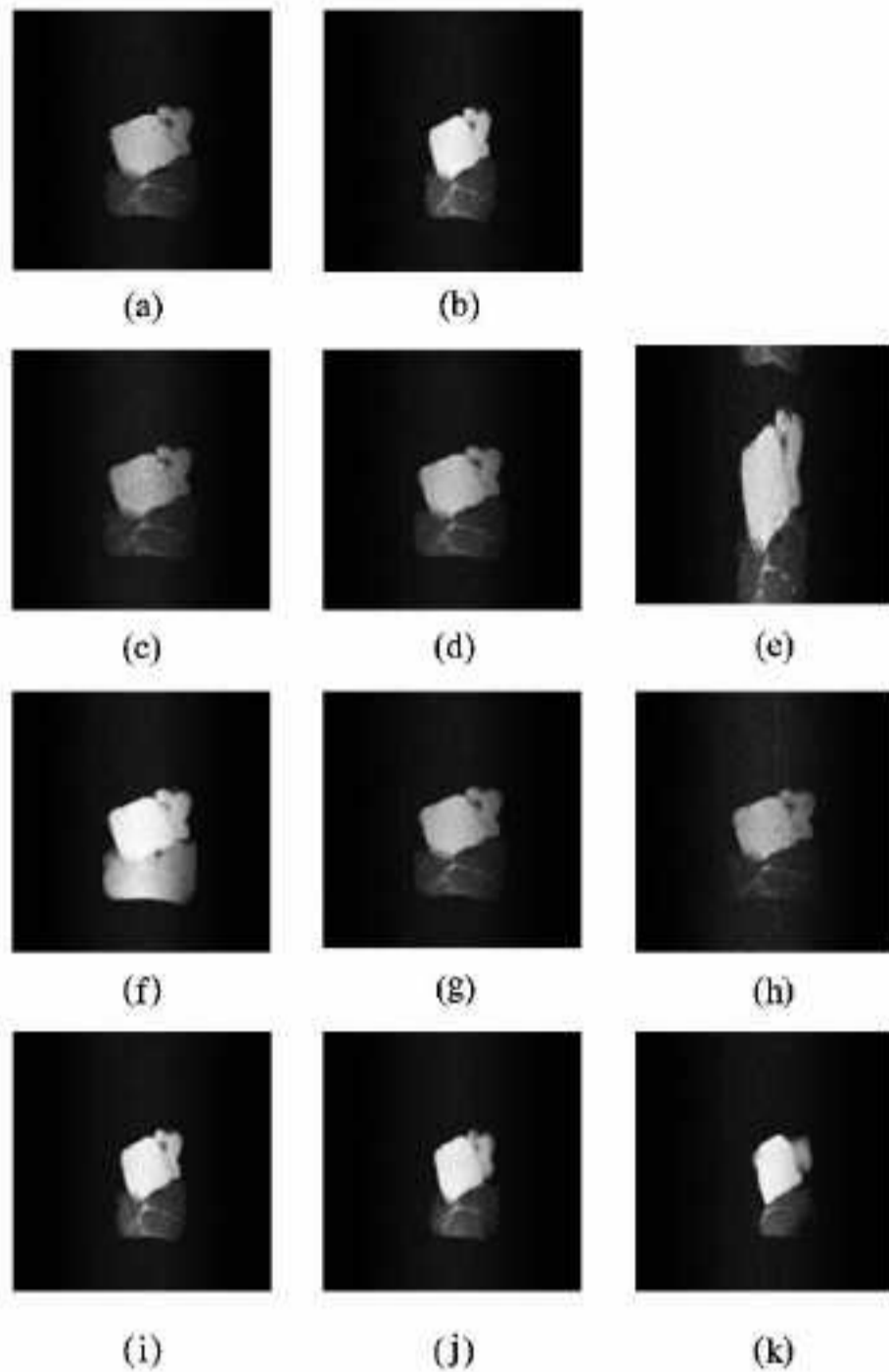
图中参数: (a-b) 选层梯度 G_x \text{ Amp} (\%) = 80, 60 ; (c-d) 累加信号次数 NS = 4, 8 ; (e) 卷褶伪影; (f-h) 序列重复时间 D_0 = 1000 \text{ ms}, 200 \text{ ms}, 50 \text{ ms} ; (i-k) 切片位置 \text{SlicePos} = +0.2 \text{ mm}, +2 \text{ mm}, +5 \text{ mm} .
