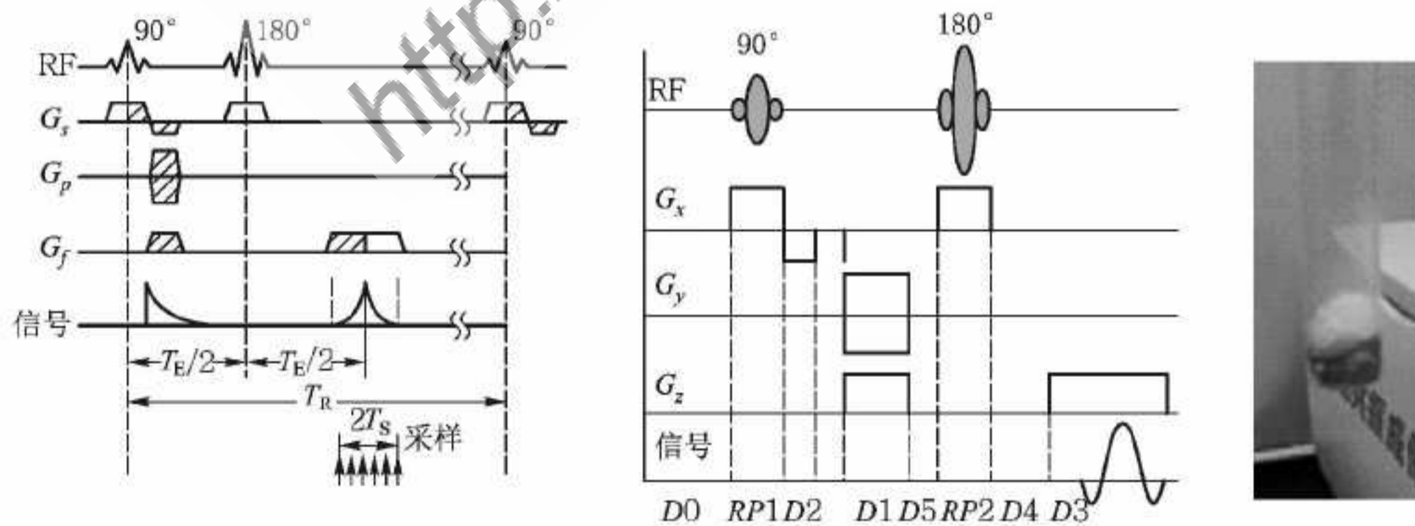
(a) 自旋回波序列示意图
