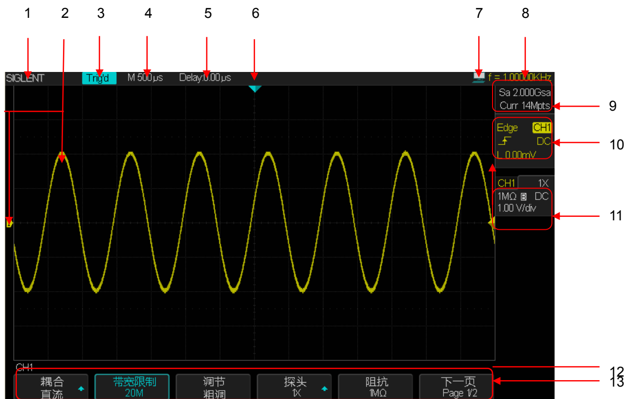
图 11 用户界面
