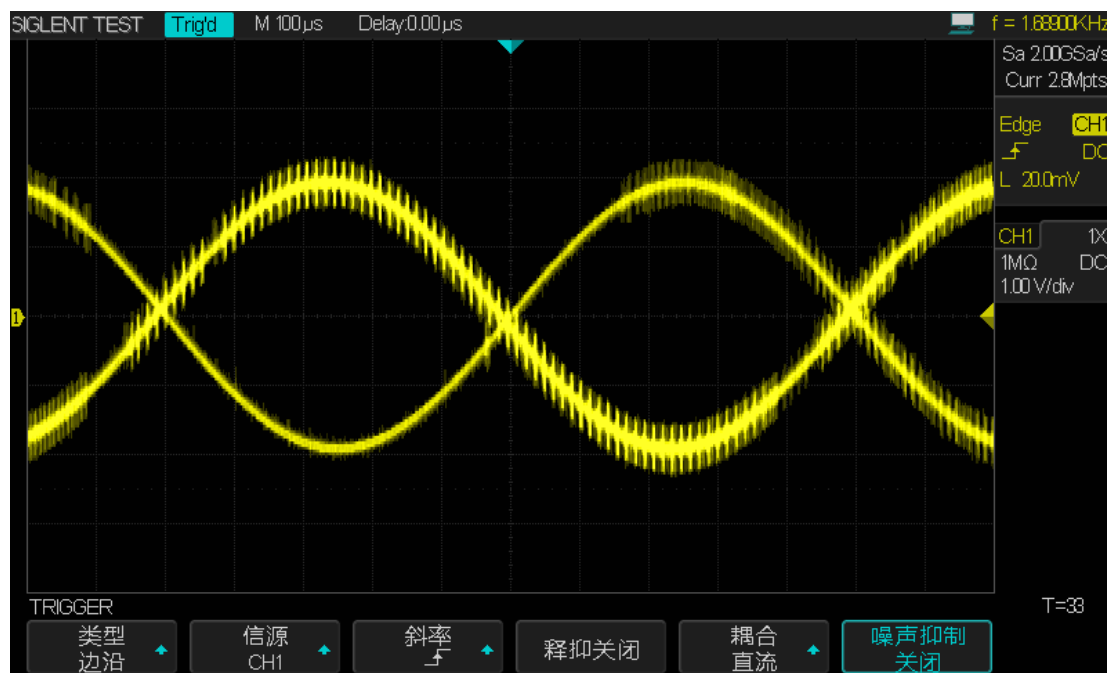
图 34 显示噪声（噪声抑制关闭）
