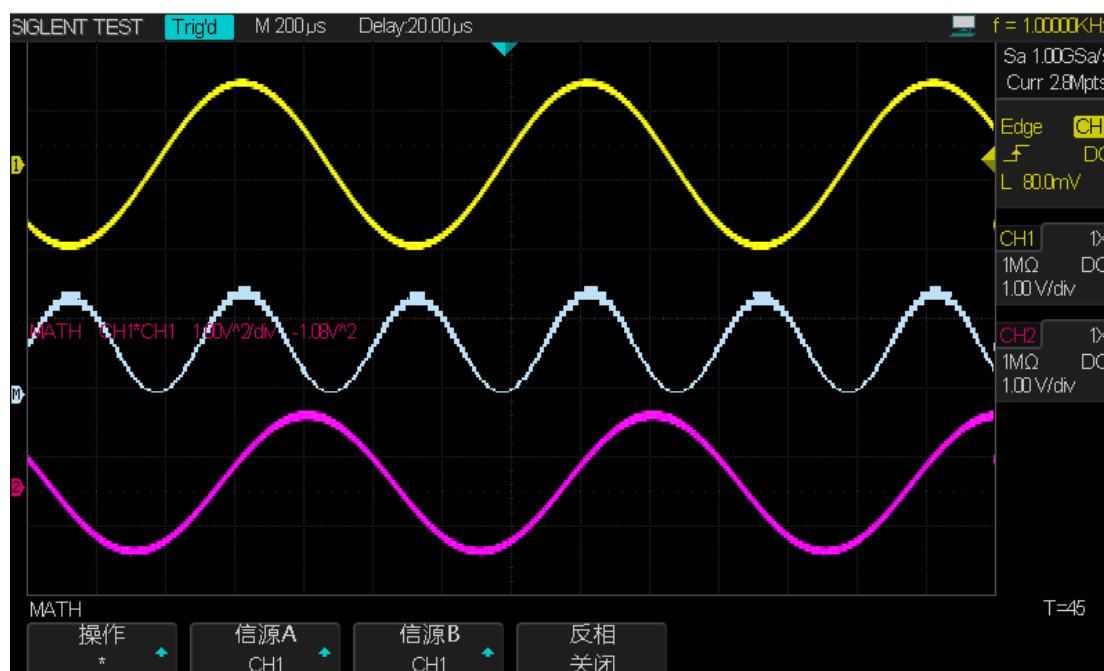
图 76 （通道 1 波形乘以通道 2 波形）
