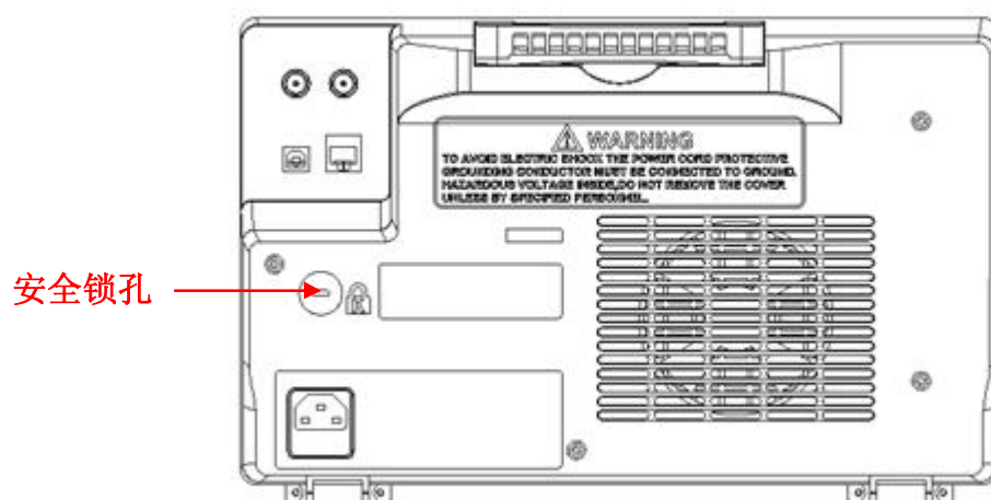
图 12 使用安全锁
