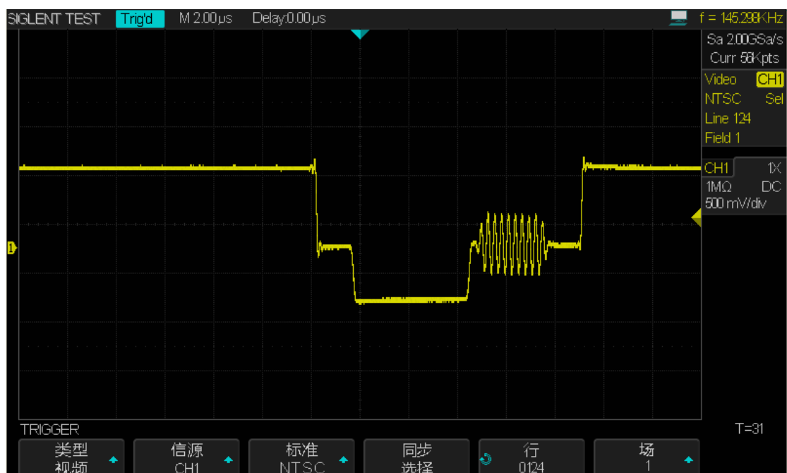
图 39 特定行上视频触发
