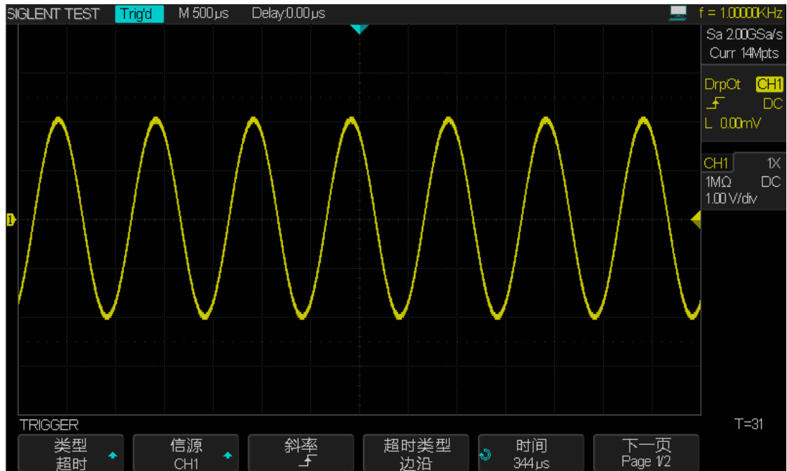
图 44 超时触发 2
