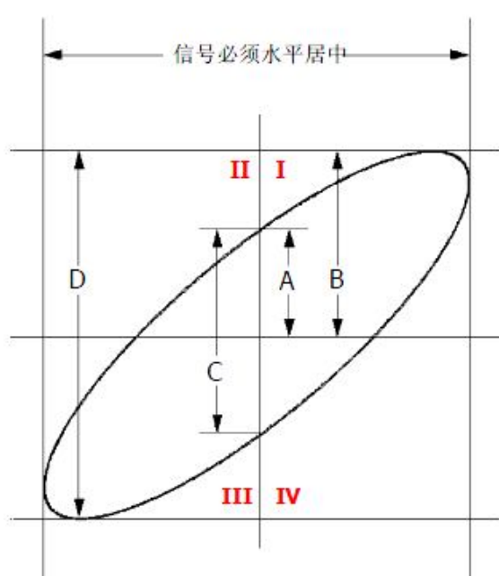
图 18 李沙育测量原理图
