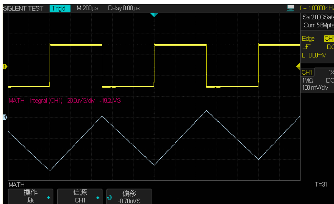
图 81 有 DC 偏移校正（积分运算）
