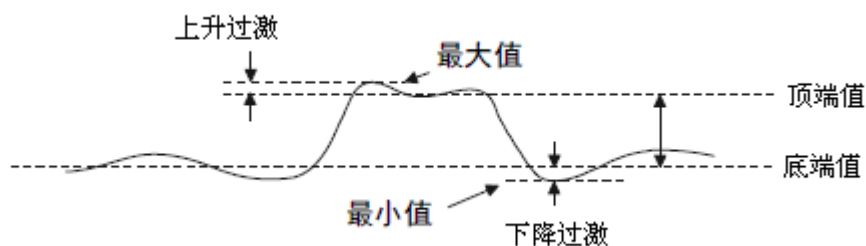
图 87 上升/下降过激示例图
