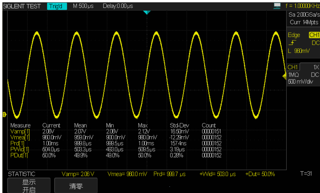
图 92 测量统计
