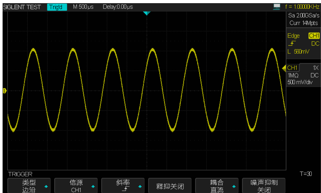
图 36 边沿触发
