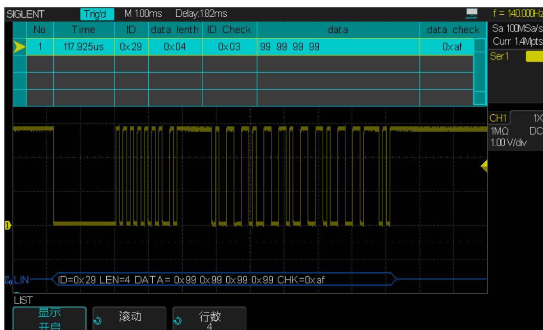
图 73 LIN 解码
