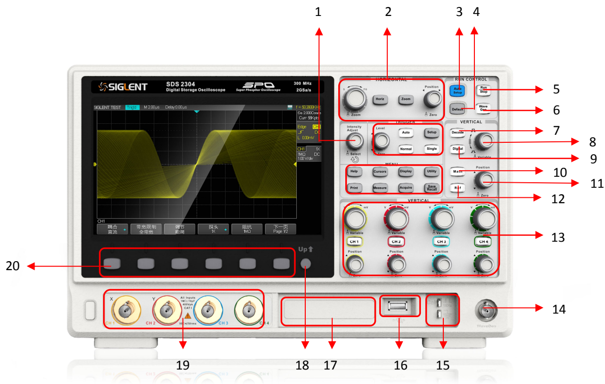
图 6 前面板总览
