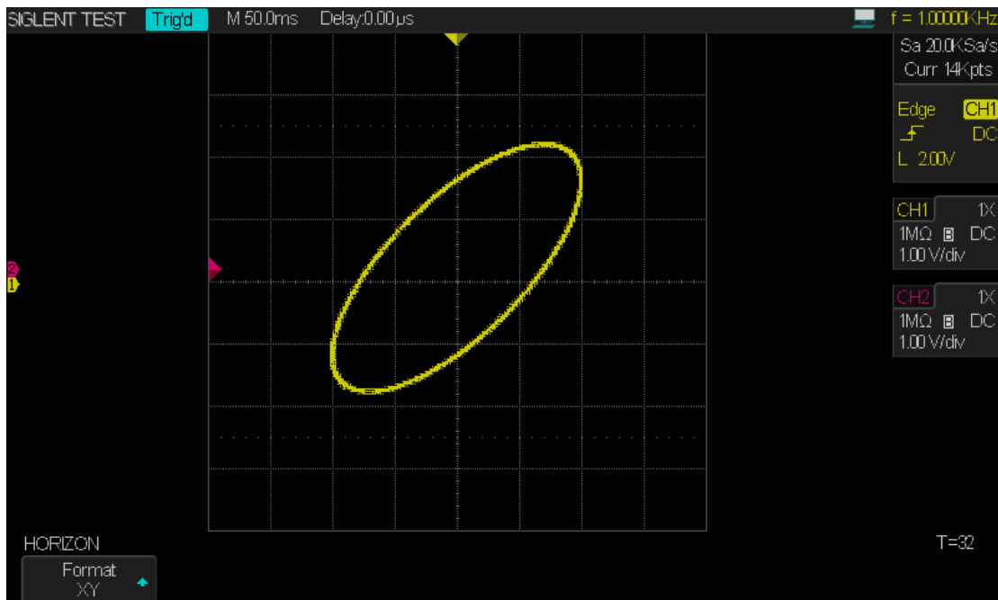
图 19 李沙育测量实例
