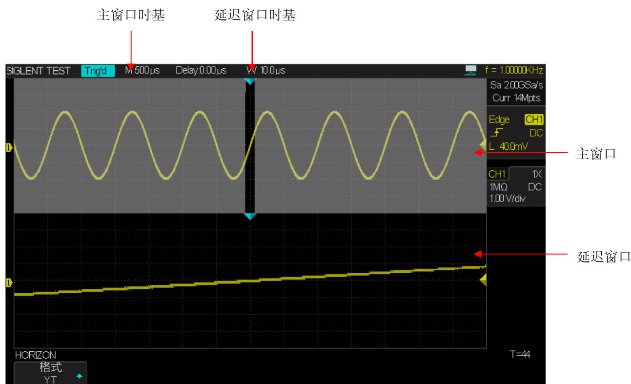
图 20 延迟扫描
