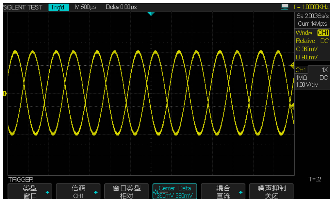
图 41 “相对”窗口触发
