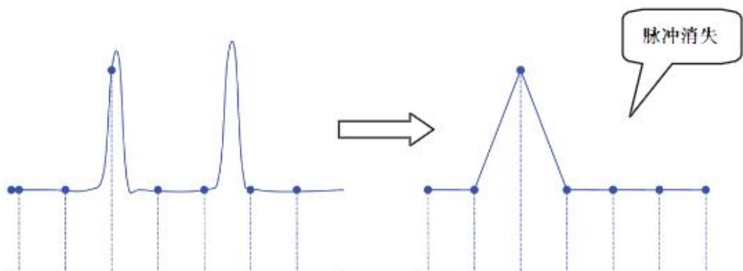
图 26 波形漏失
