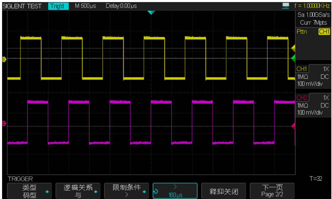
图 51 码型触发 2 (2/2 页)
