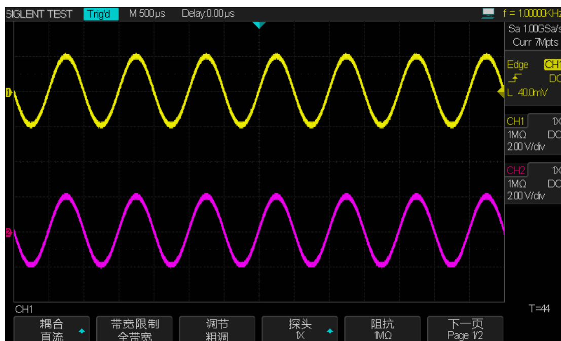
图 14 通道波形图
