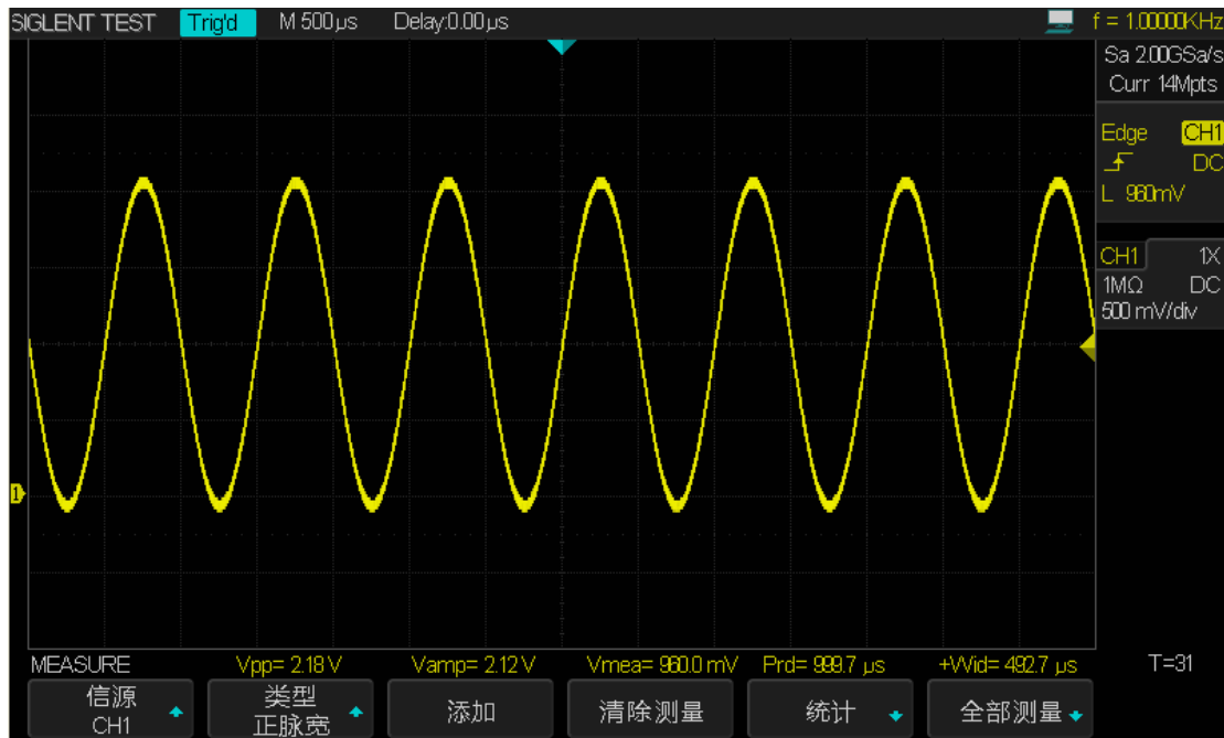
图 90 自动测量图 1（5 个参数）
