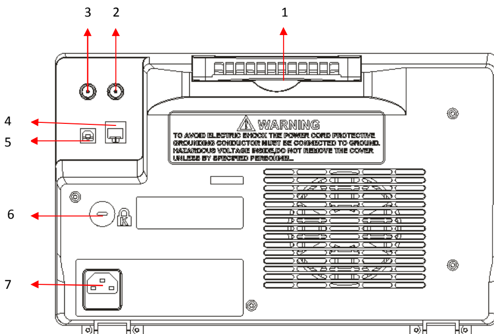
图 7 后面板总览
