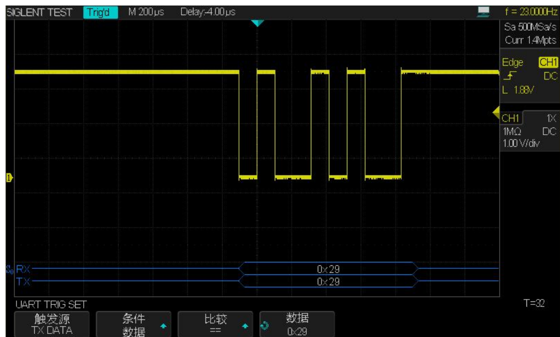
图 66 UART 触发
