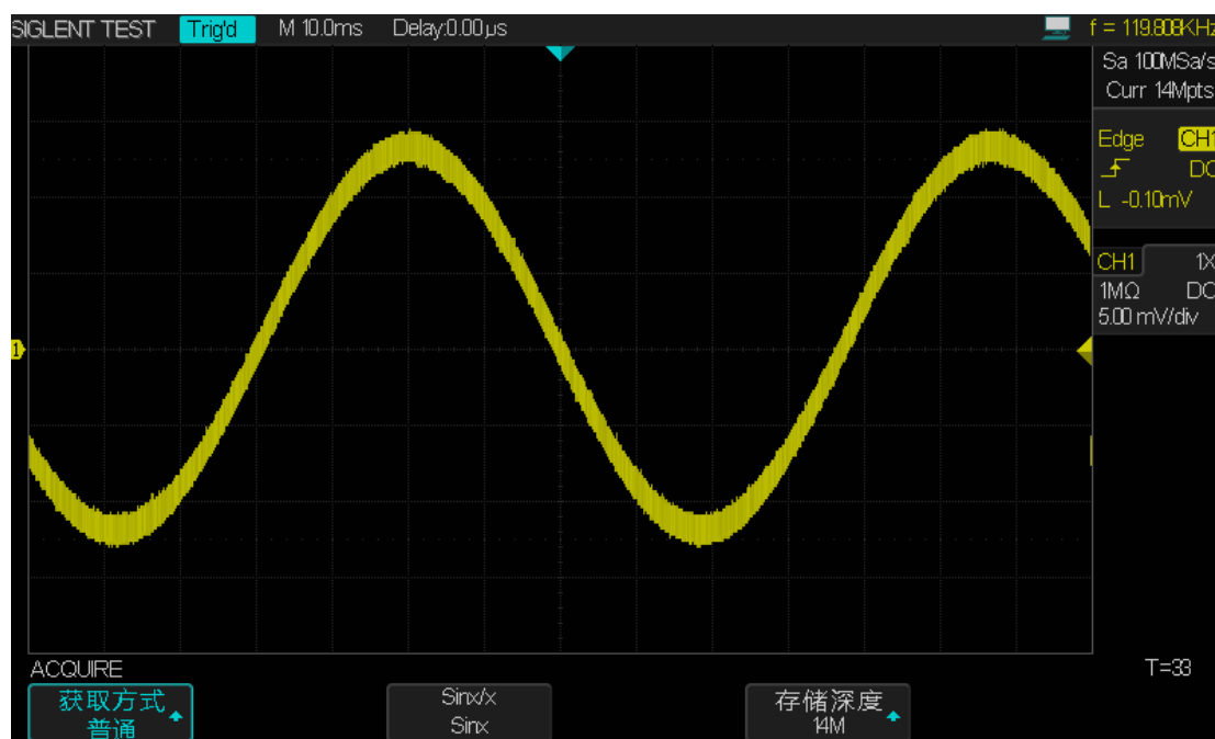
图 31 未平均时的波形（显示波形上的随机噪声）
