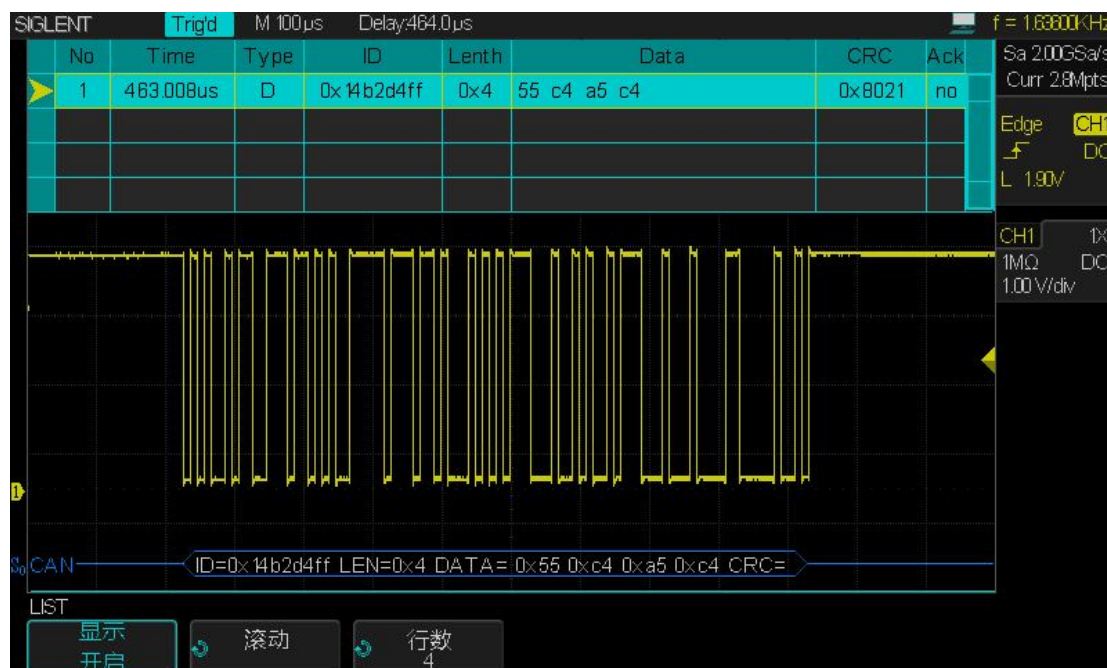
图 70 CAN 解码
