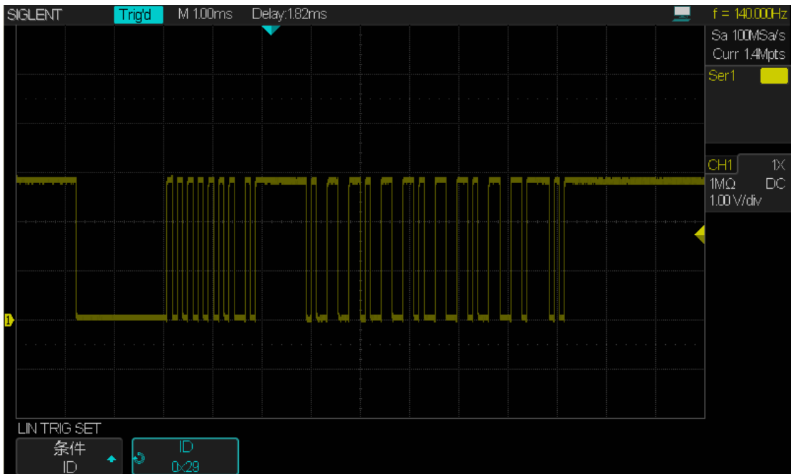
图 72 LIN 触发
