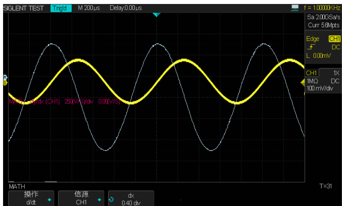
图 79 微分运算
