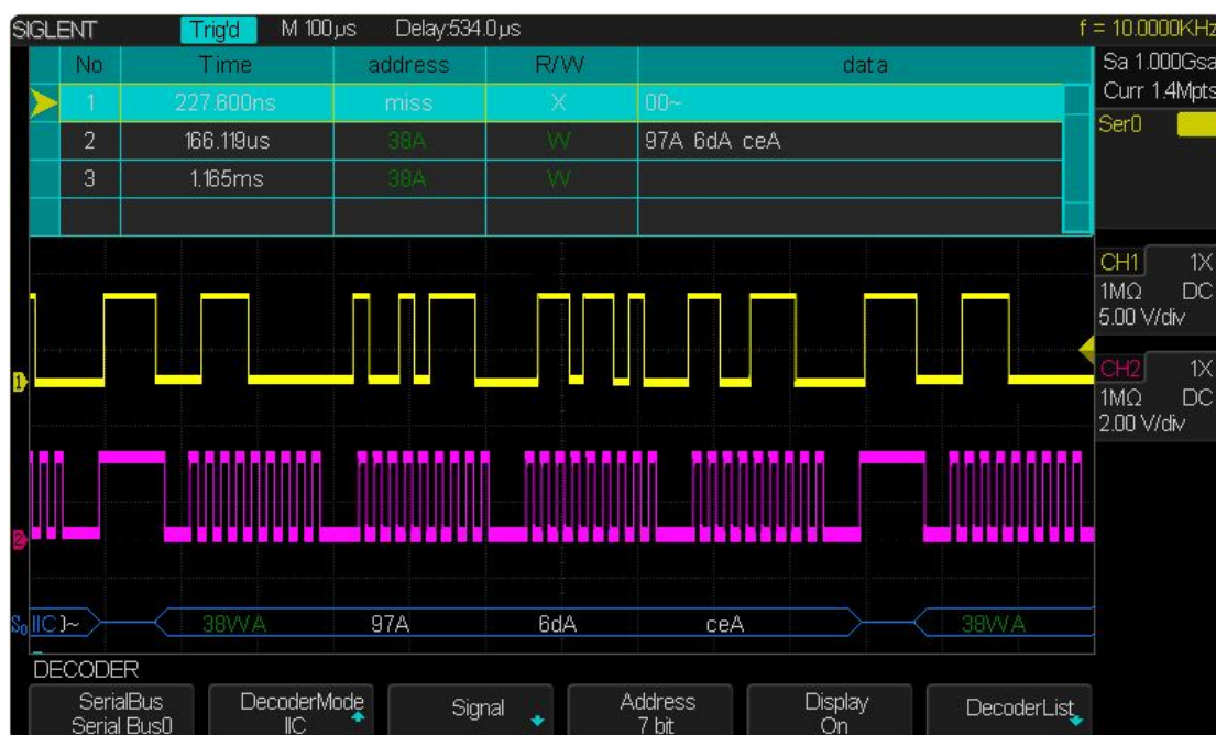
图 55 IIC 解码图
