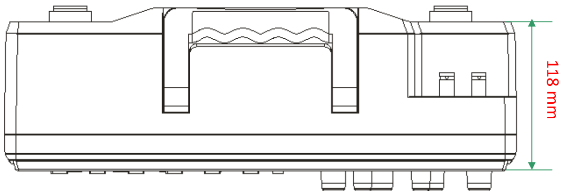
图 2 侧视图
