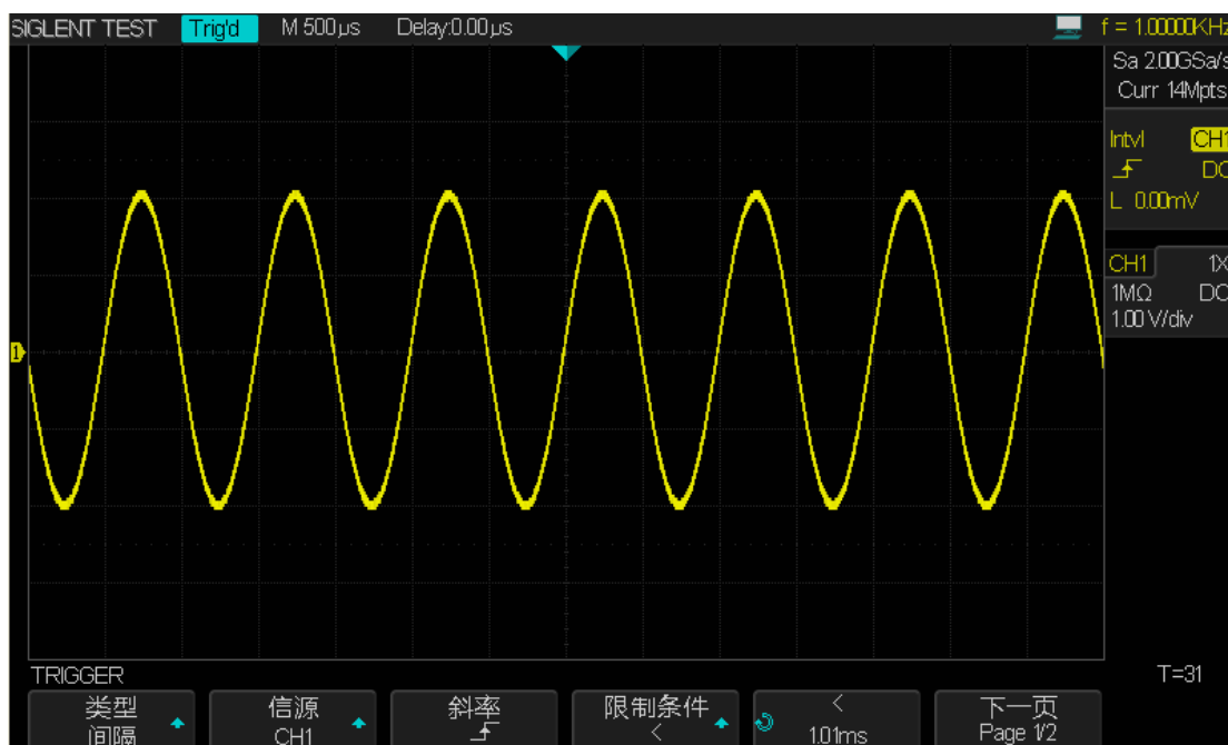
图 43 超时触发 1
