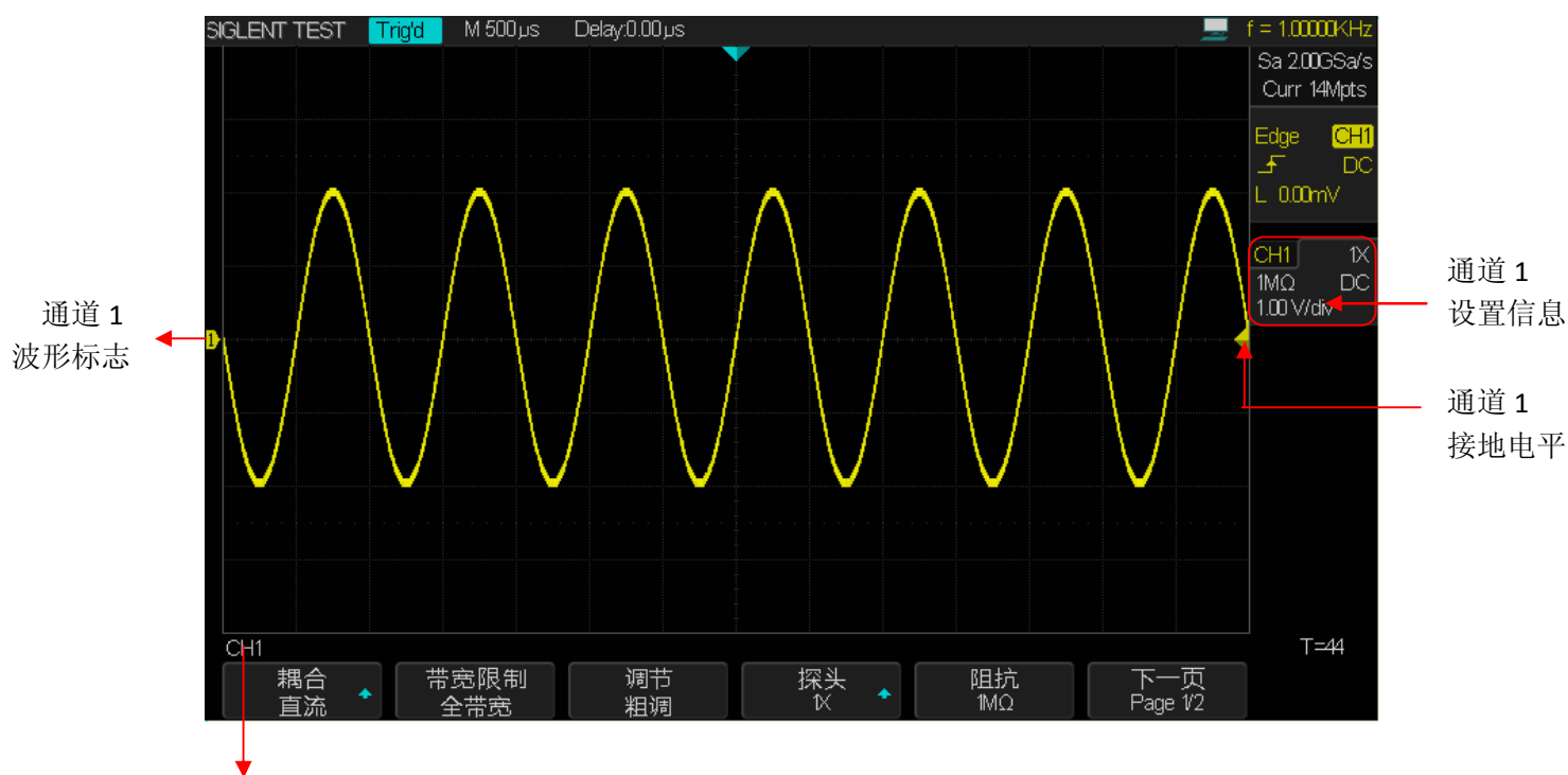
图 13 垂直通道图
