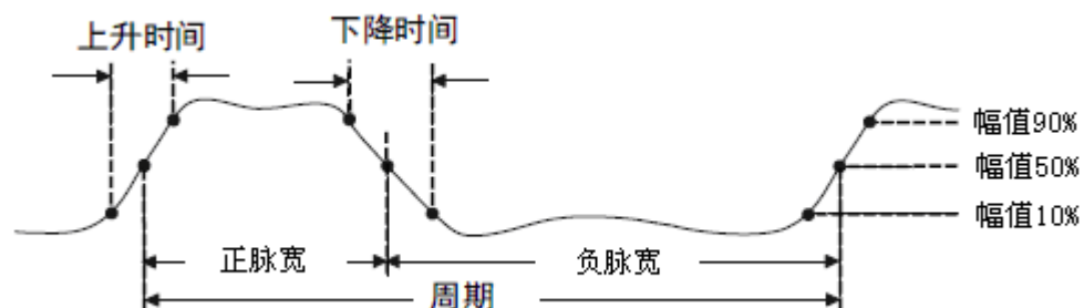
图 89 时间参数示意图
