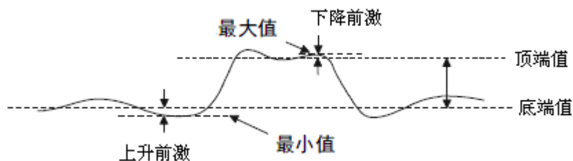
图 88 上升/下降前激
