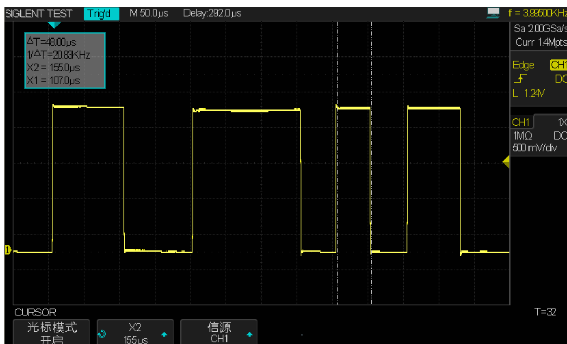
图 83 脉冲宽度测量
