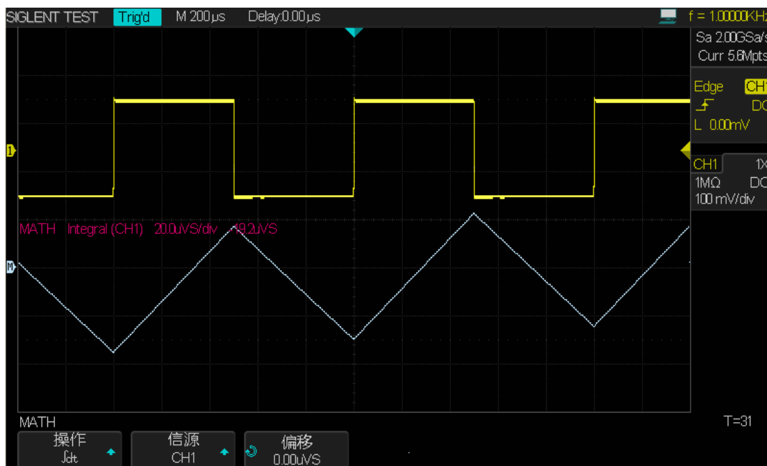
图 80 无 DC 偏移校正（积分运算）
