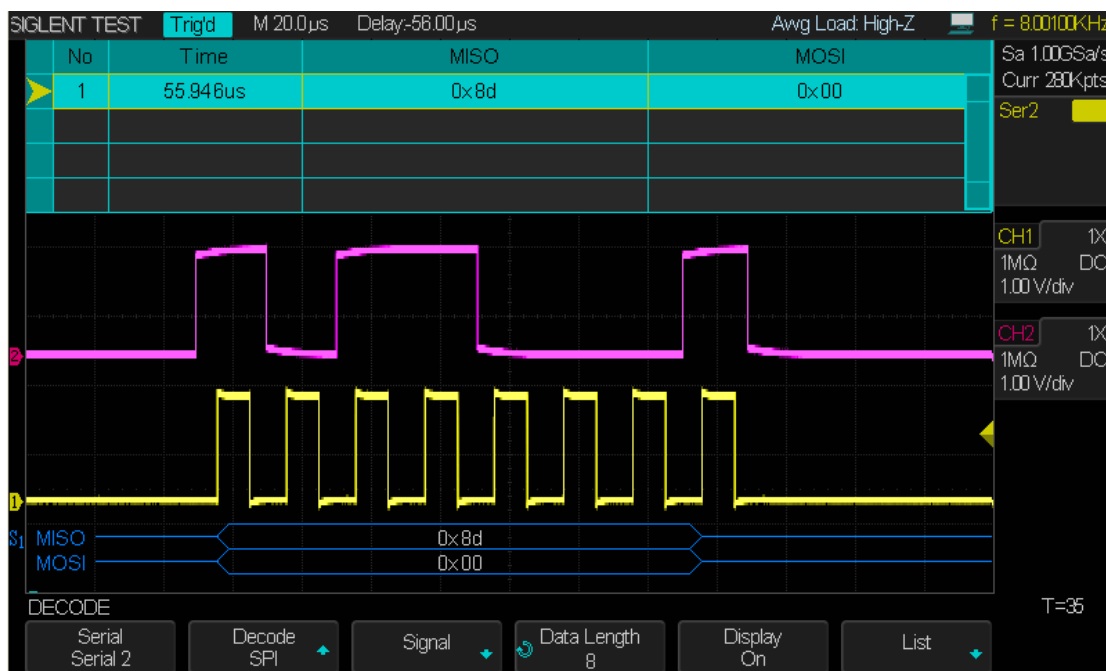
图 62 SPI 解码图
