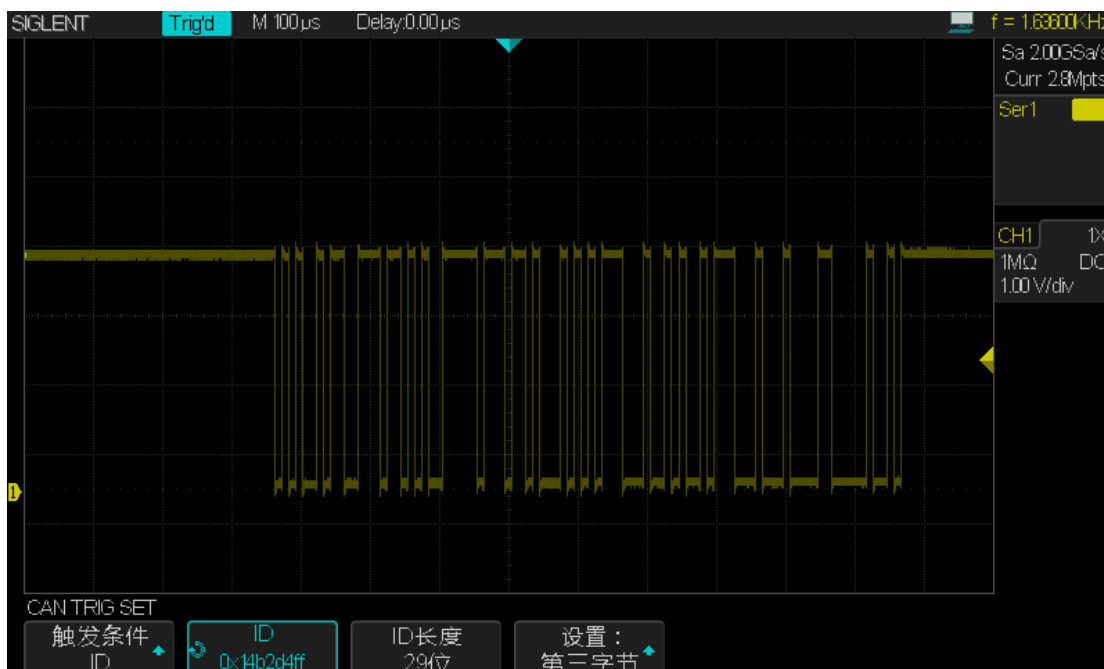
图 69 CAN 触发
