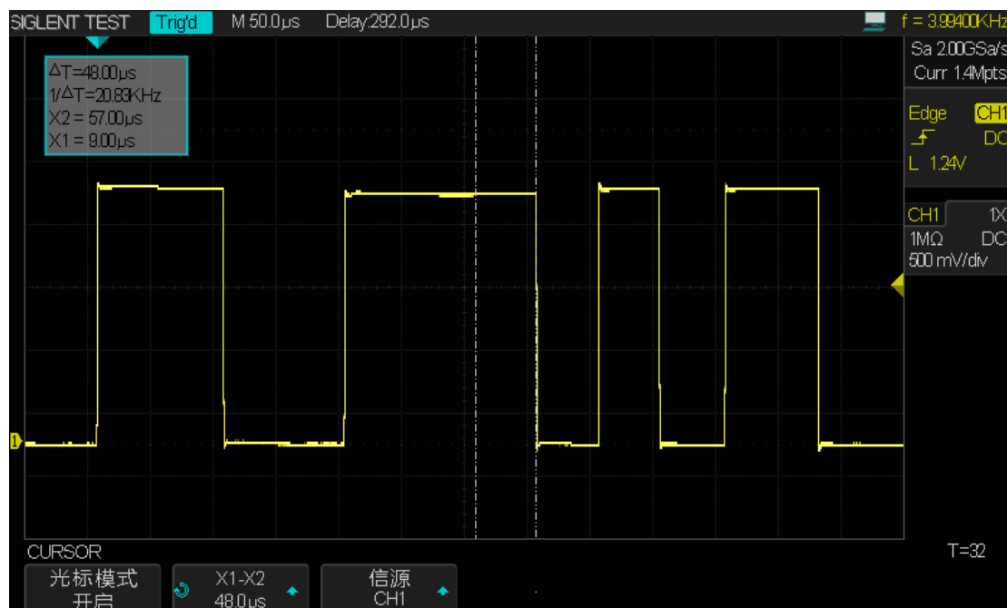
图 84 脉宽变化检测
