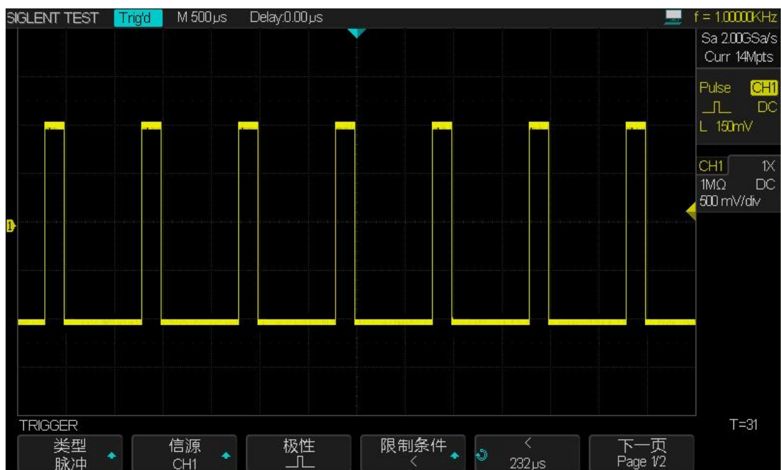
图 38 脉冲触发
