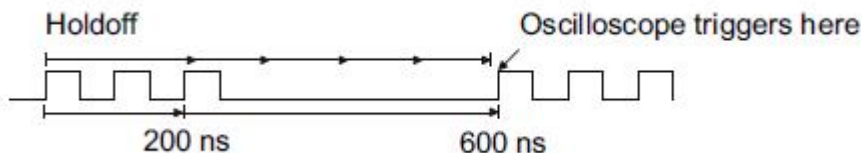
图 33 设置触发释抑时间
