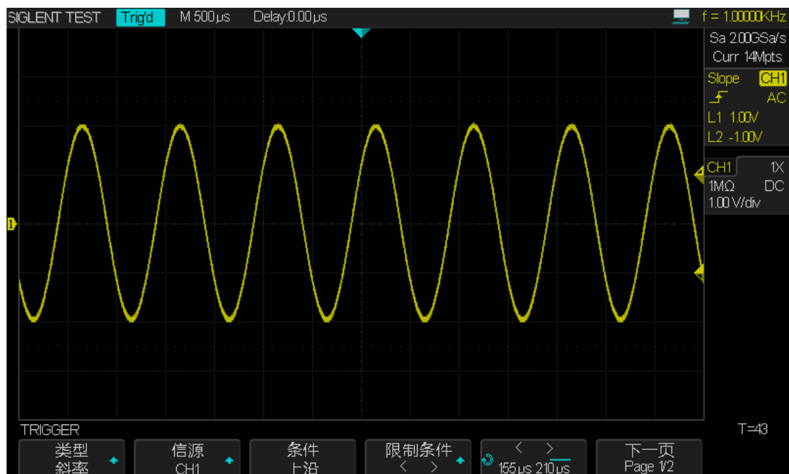
图 37 斜率触发
