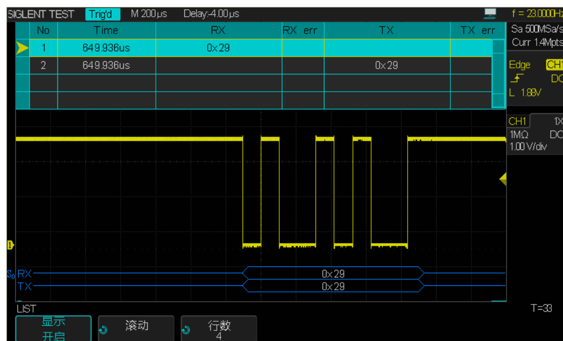
图 67 UART 解码
