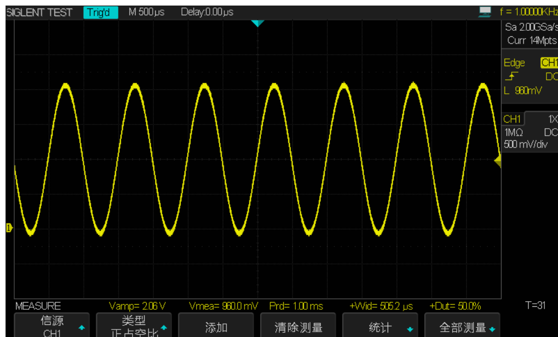
图 91 自动测量图 2（添加“+Dut”）
