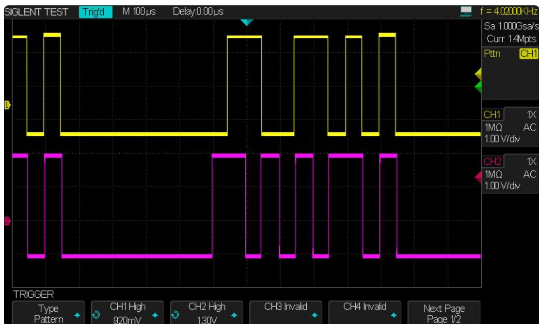
图 48 码型触发 1 (1/2 页)
