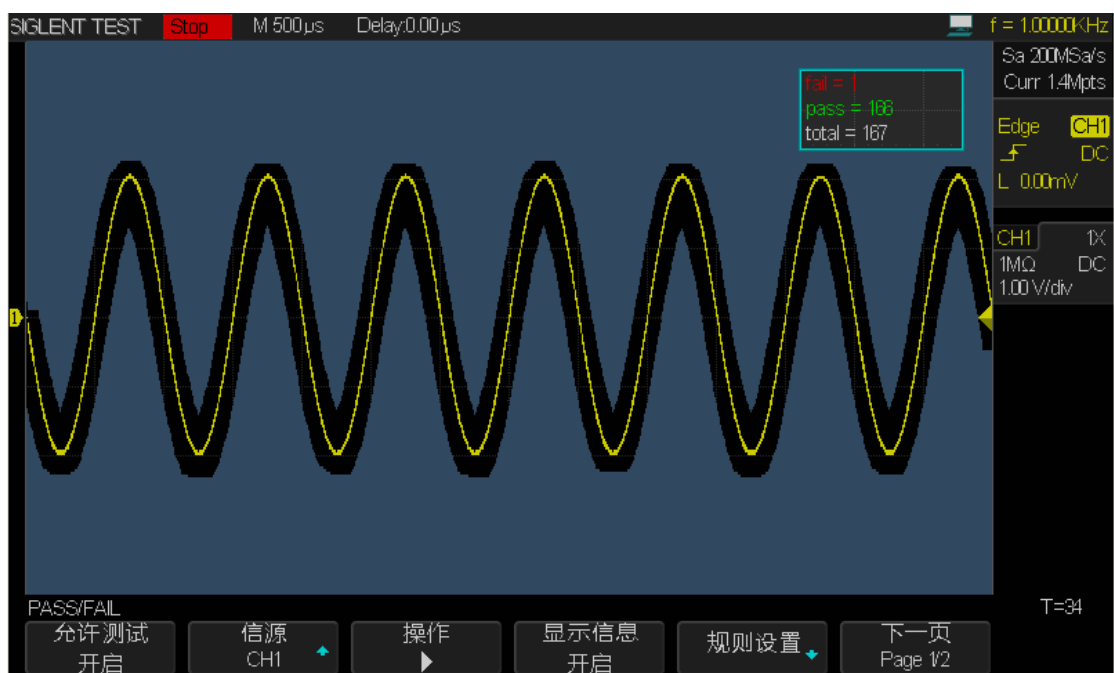
图 113 检测到失败脉冲
