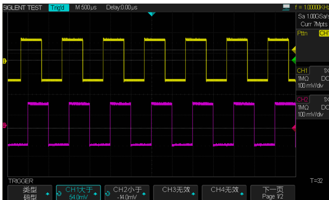
图 50 码型触发 2 (1/2 页)
