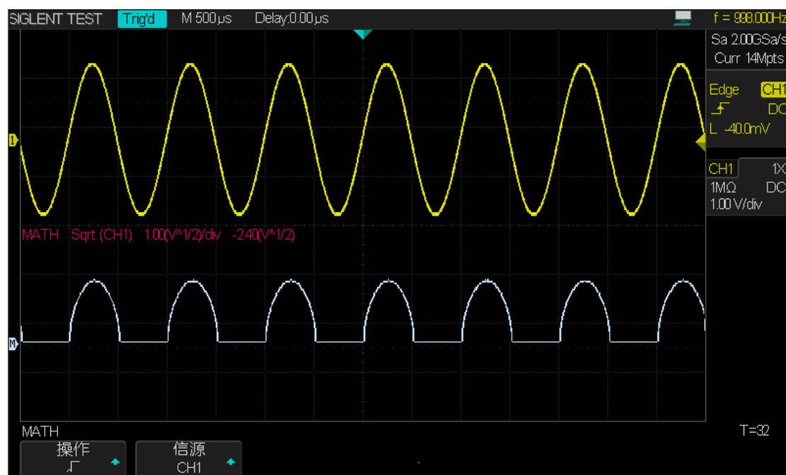
图 85 峰峰值测量
