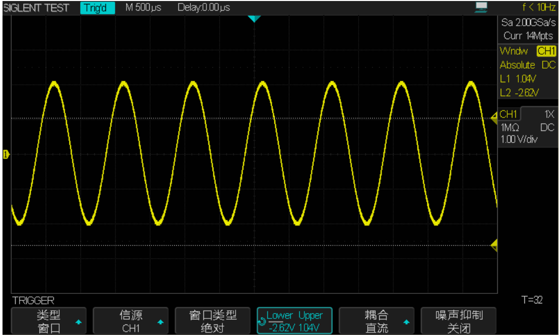
图 40 “绝对”窗口触发
