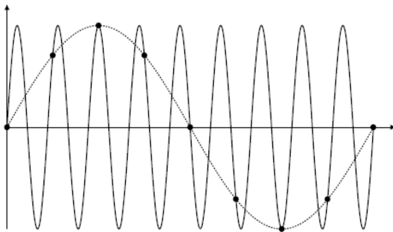
图 21 采样混叠
