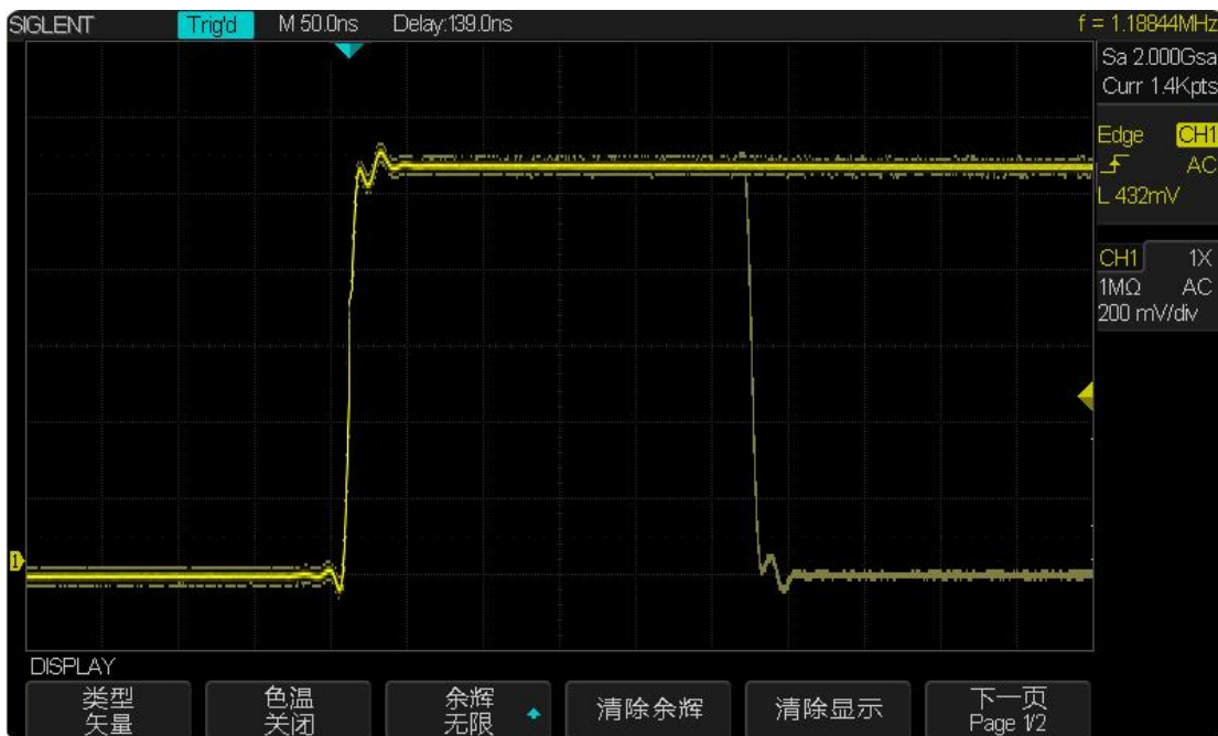
图 97 用“无限”余辉捕捉异常信号
