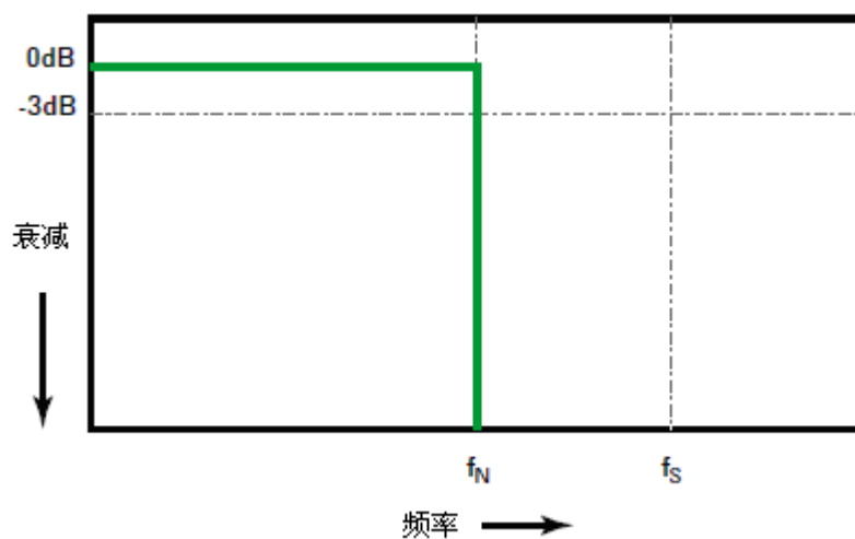
图 22 理论上的砖墙频率响应
