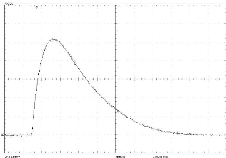
弱辐射时的完整脉冲
