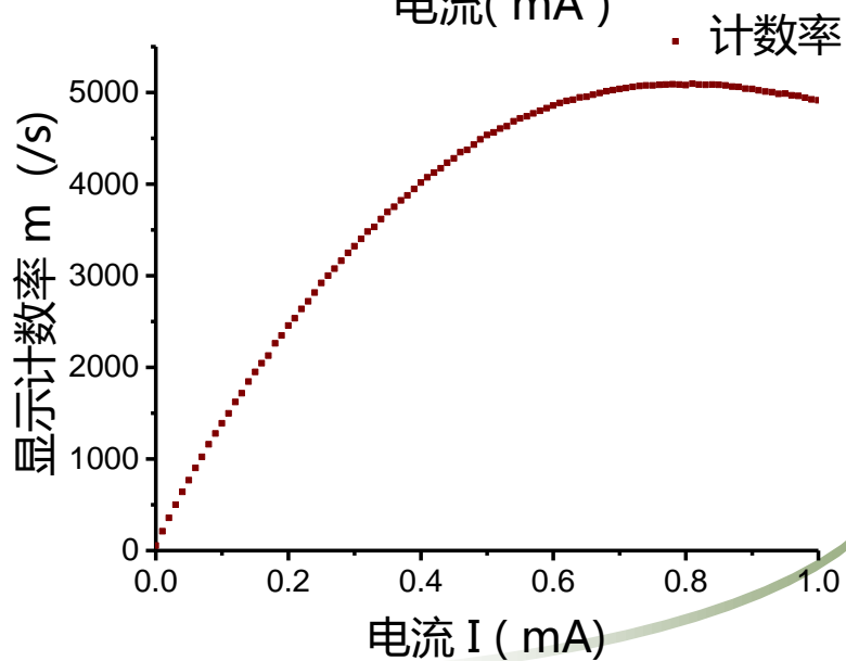
管端电压为417V下的计数结果
