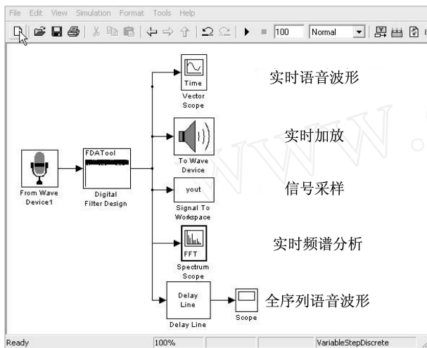
图 1 simulink 数据采集面板
