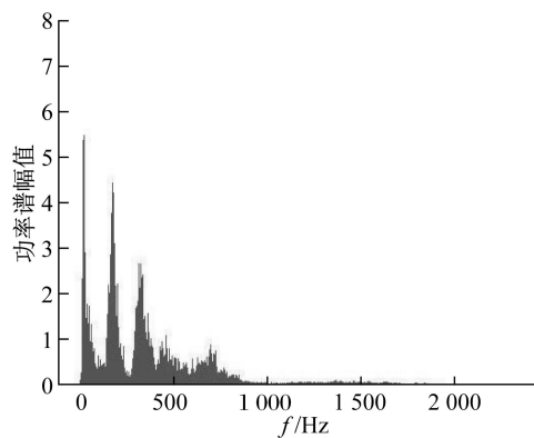
图 2 发声频谱
