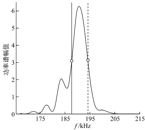
图 4 低频半峰宽
