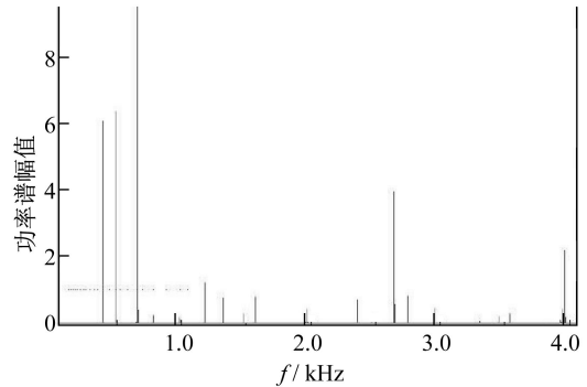
图 7 定音器频谱
