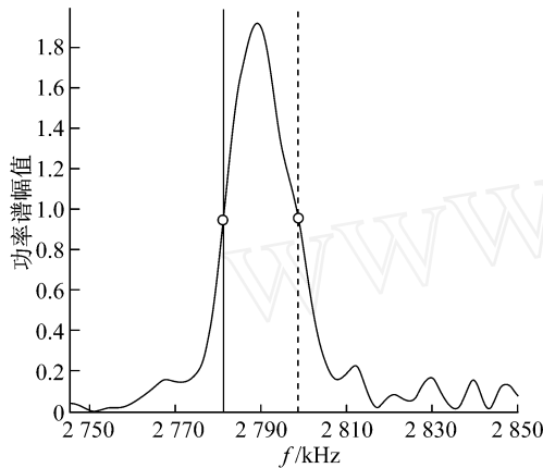
图 4 低频半峰宽
