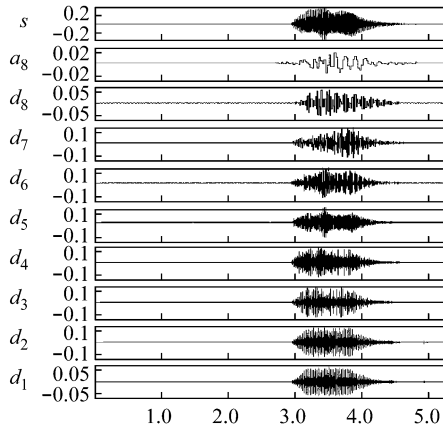
图 9 小波分解系数图
