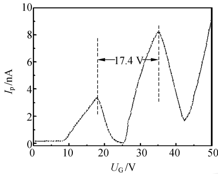
图 2 I-U 曲线
