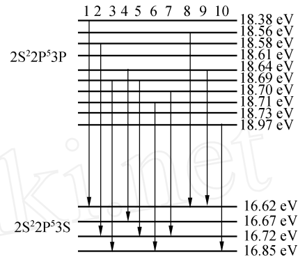
图 5 实验中测量的光谱对应的能级跃迁
